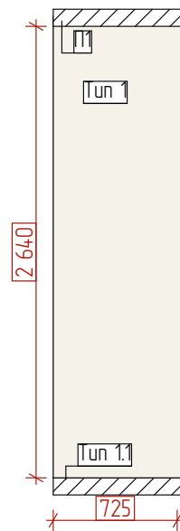
01 Вид 01:40
