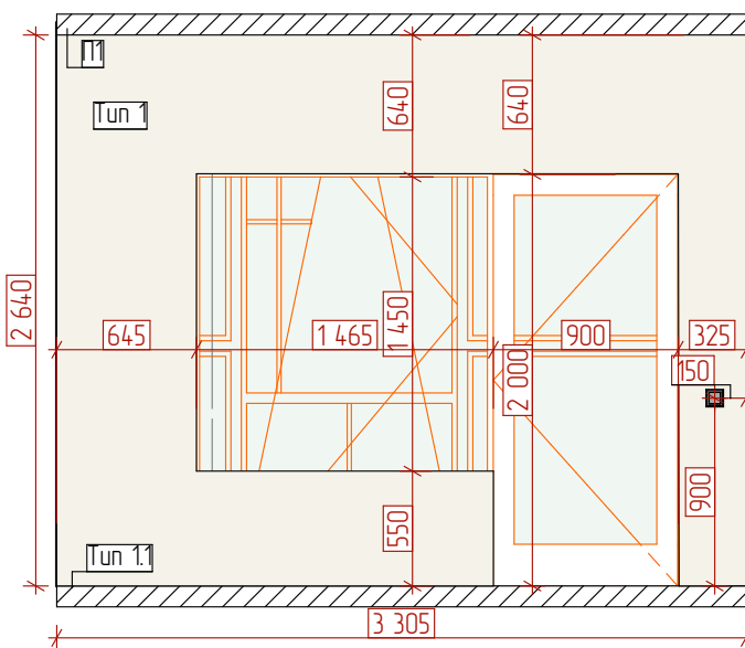
05 Вид 05 1:40
