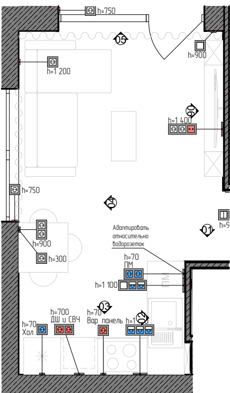
1. Кухня - гостиная 1:60
