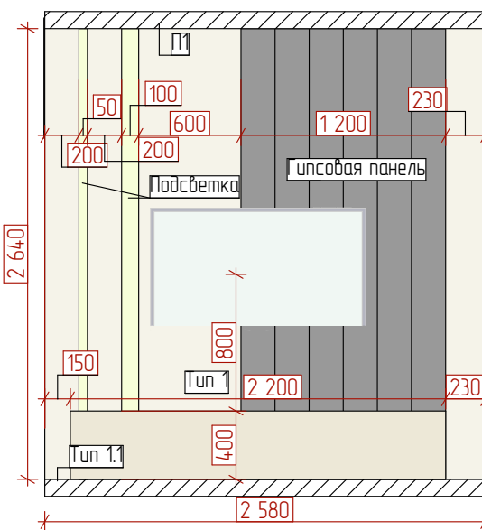
06 Вид 06 1:40
