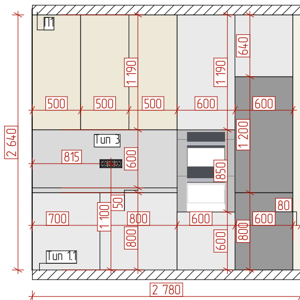
03 Вид 03 1:40
