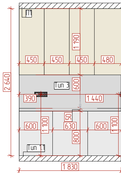
02 Вид 02 1:40
