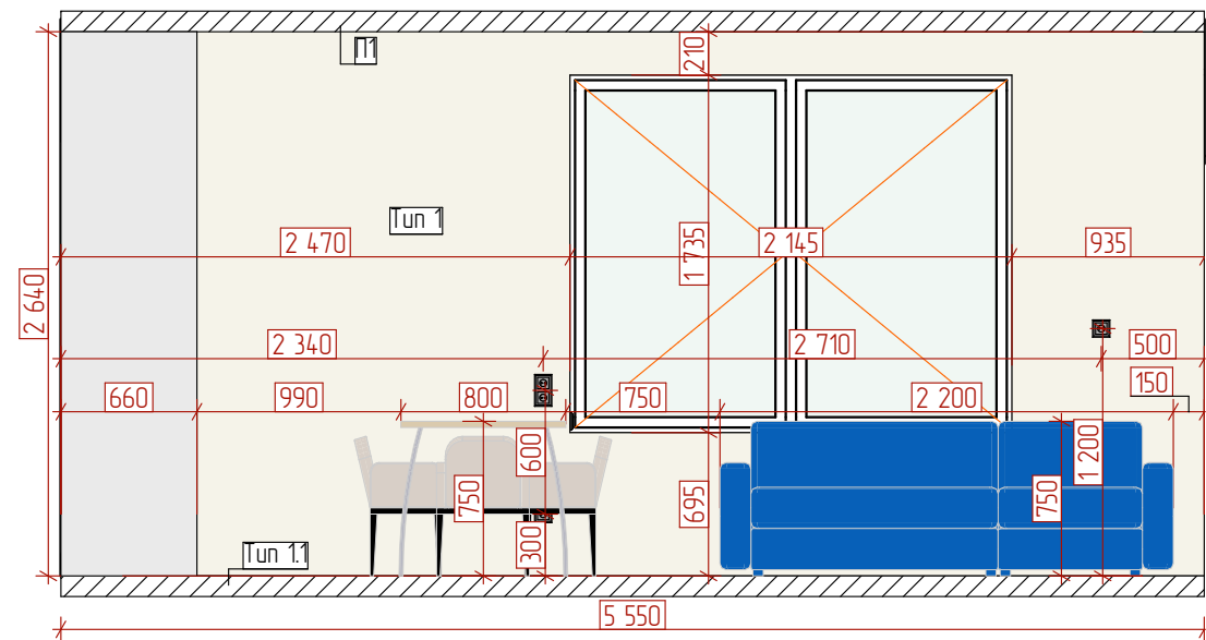
04 Вид 04 1:40
